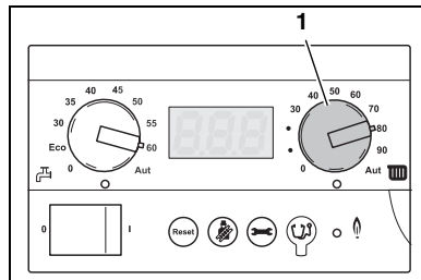
afb. 19 BC10 – cv-waterinstelling
