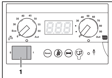
afb. 22 BC10
