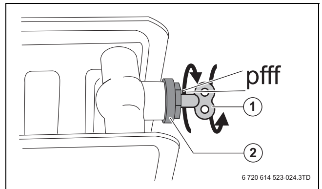
Afb. 8 Ontluchten radiator
