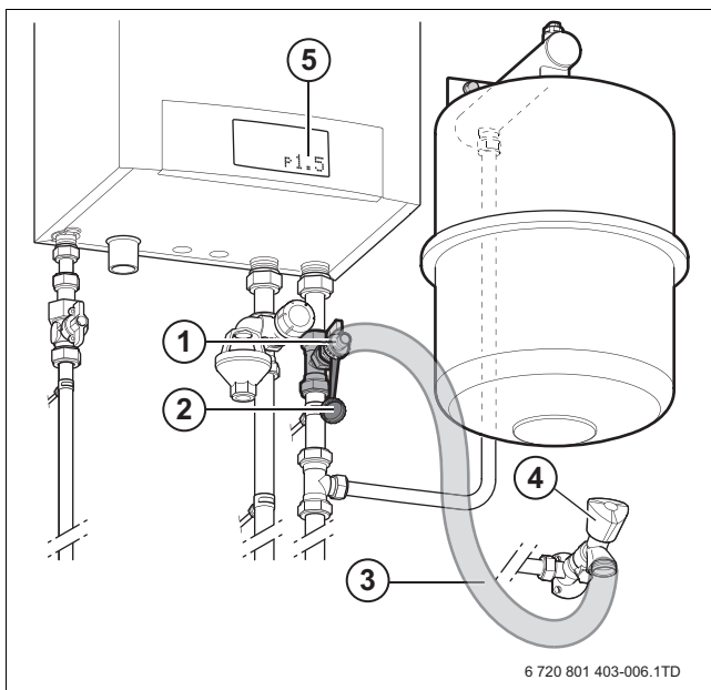
Afb. 7 Bijvullen cv-installatie
