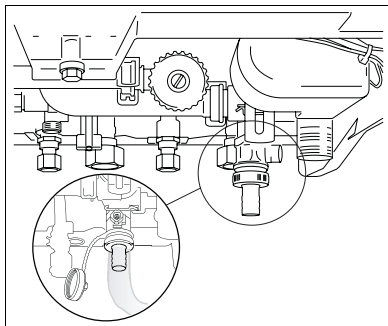
Afb. 6 Cv-installatie vullen (SmartLine HRC 24 uitgebreid)
