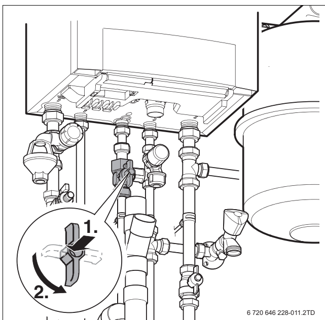
Afb. 3 Gaskraan
