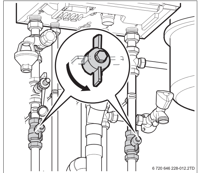
Afb. 4 Serviceafsluiters
