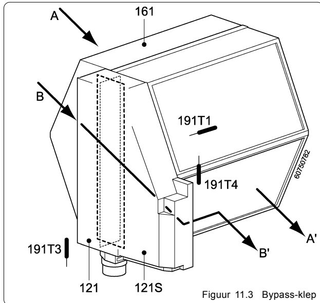
Figuur 11.3 Bypass-klep
